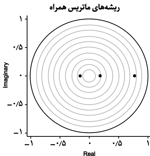
شکل ۱. ریشه‌های ماتریس و شرط پایداری
